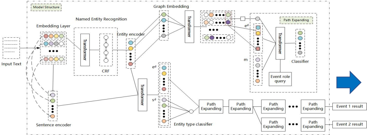
基于知识增强的事件抽取模型
